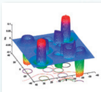
Przestrzenny rozkład stałego pola magnetycznego nad dyskiem ADR-4. Dysk wytwarza pole magnetyczne o natężeniu 30 gausów (3 militesle).
